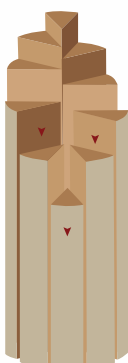
KATXS1 KATXS2
